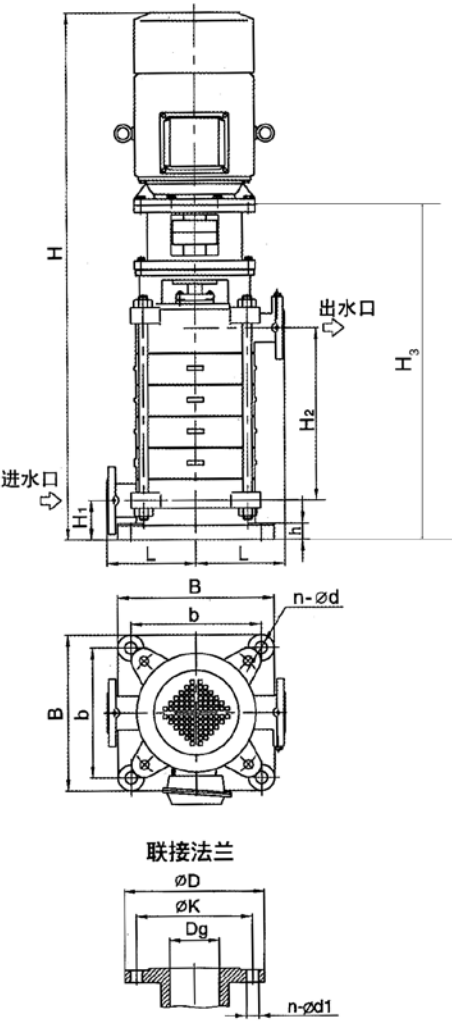
外形安装尺寸图
