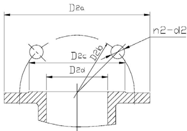
出口法兰
