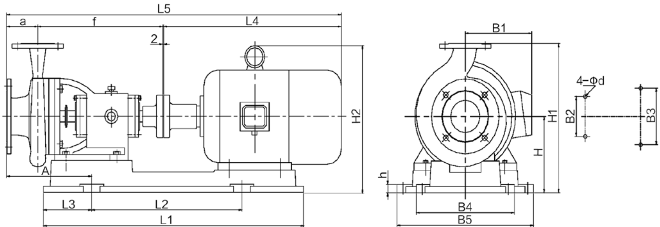
FT系列泵外形安装尺寸图
