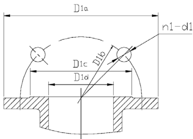
进口法兰
