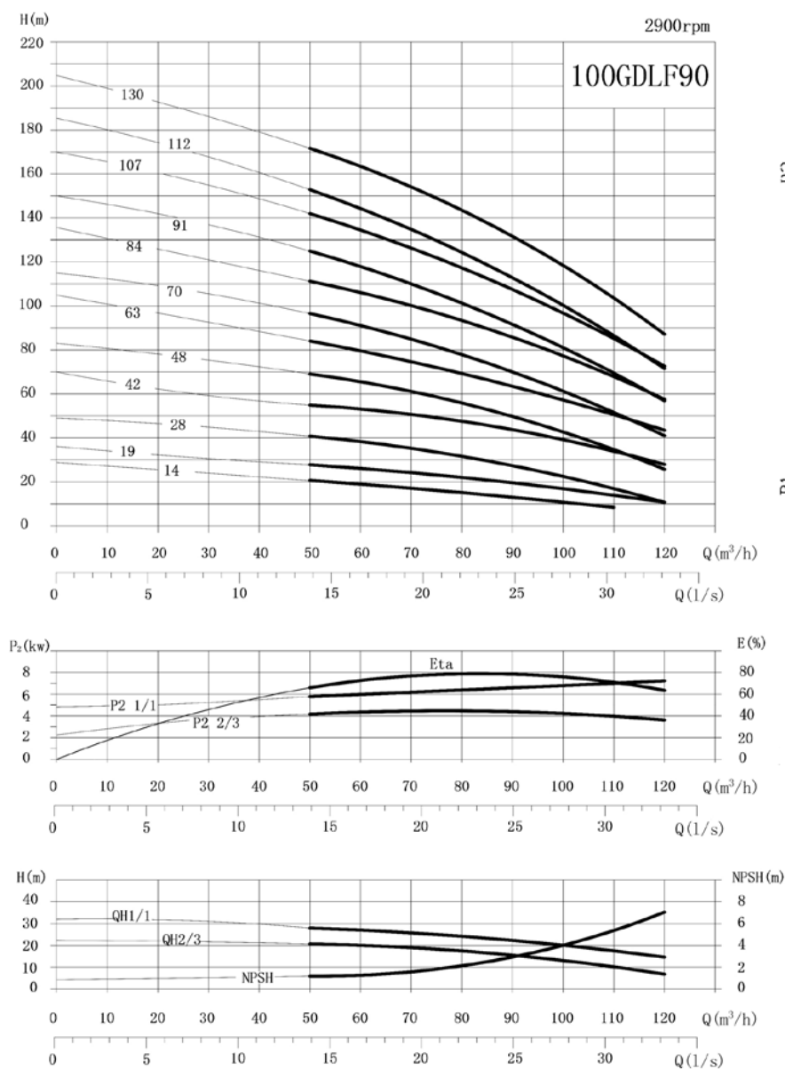
性能曲线 CURVES
